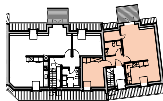
2. Salsplan 2 rums lejlighed
